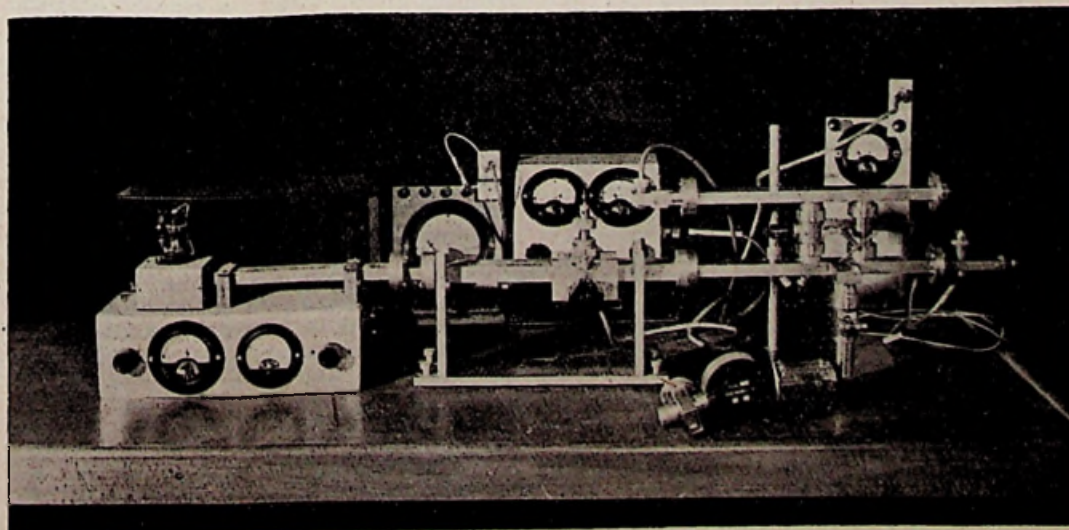
De Telecommunicatie-Industrie te Hilversum houdt zich natuurlijk ook met radar bezig. De foto laat ons een gedeelte zien van een proefopstelling voor radar in het laboratorium. Op de voorgrond een zgn. Magnetron.
